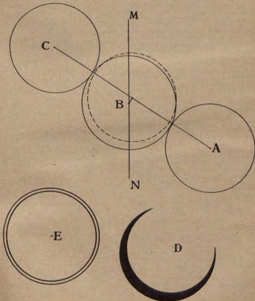
Zaćmienie słońca d. 17 kwietnia 1912 r. Przebieg zjawiska, obserwowanego w Warszawie.
