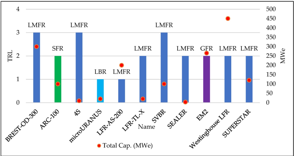
Rys. 6. Poziom TRL dla reaktorów wykorzystujących neutrony prędkie [15]. Fig. 6. TRL for fast neutrons reactors [15].
