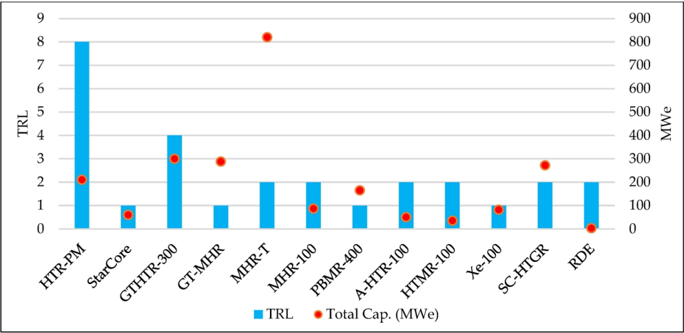
Rys. 5. Ocena poziomu TRL dla HTGR SMR [15]. Fig. 5. Evaluation of TRL for HTGR SMR [15].
