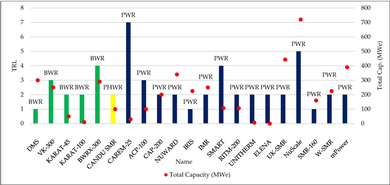
Rys. 4. Ocena poziomu TRL dla wybranych SMR [15]. Fig. 4. Evaluation of TRL for selected SMRs [15].
