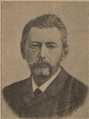
Józef Bliziński
